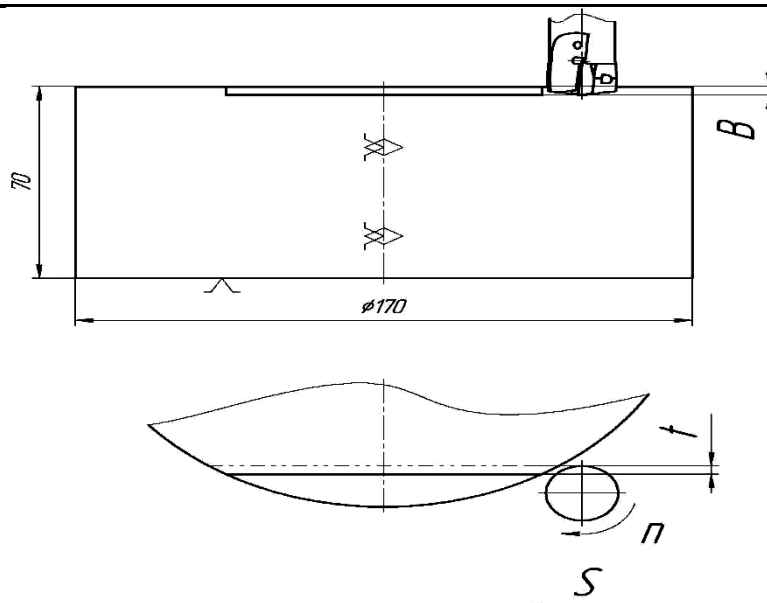
2-расм. Барқарорлик синовларида қуйим кесиш схемаси.
