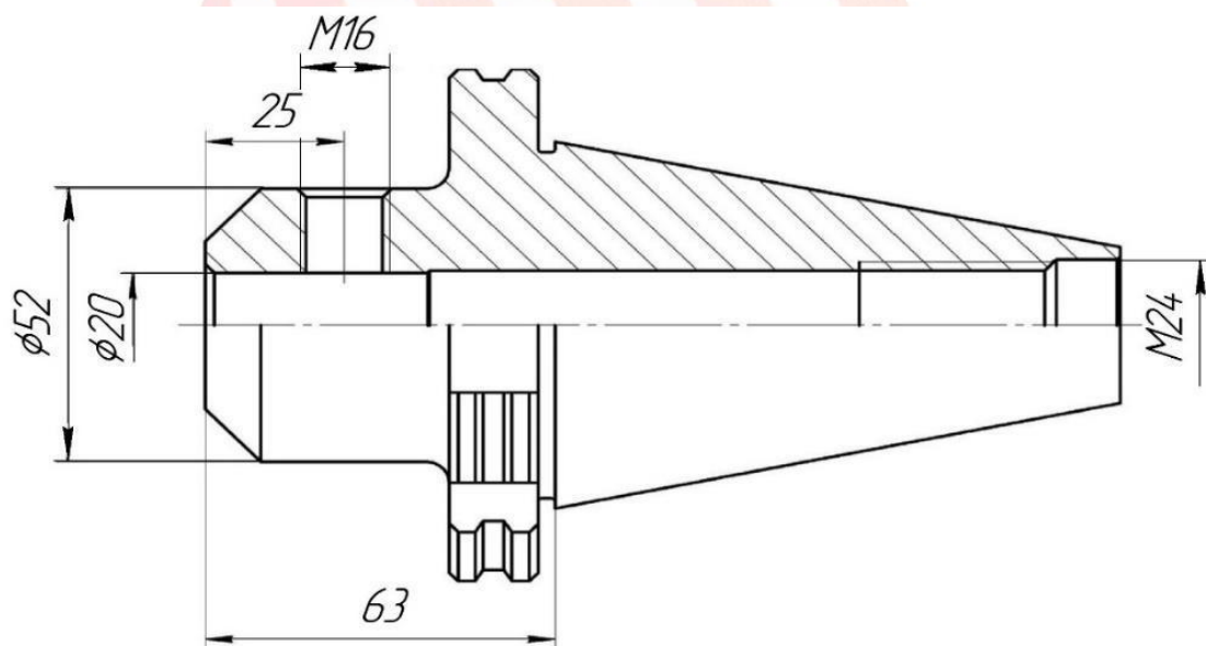
3 – расм. Weldon SK50-SLA20-63 патрони
